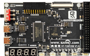
VF-T20F256 Trion入门FPGA开发板
